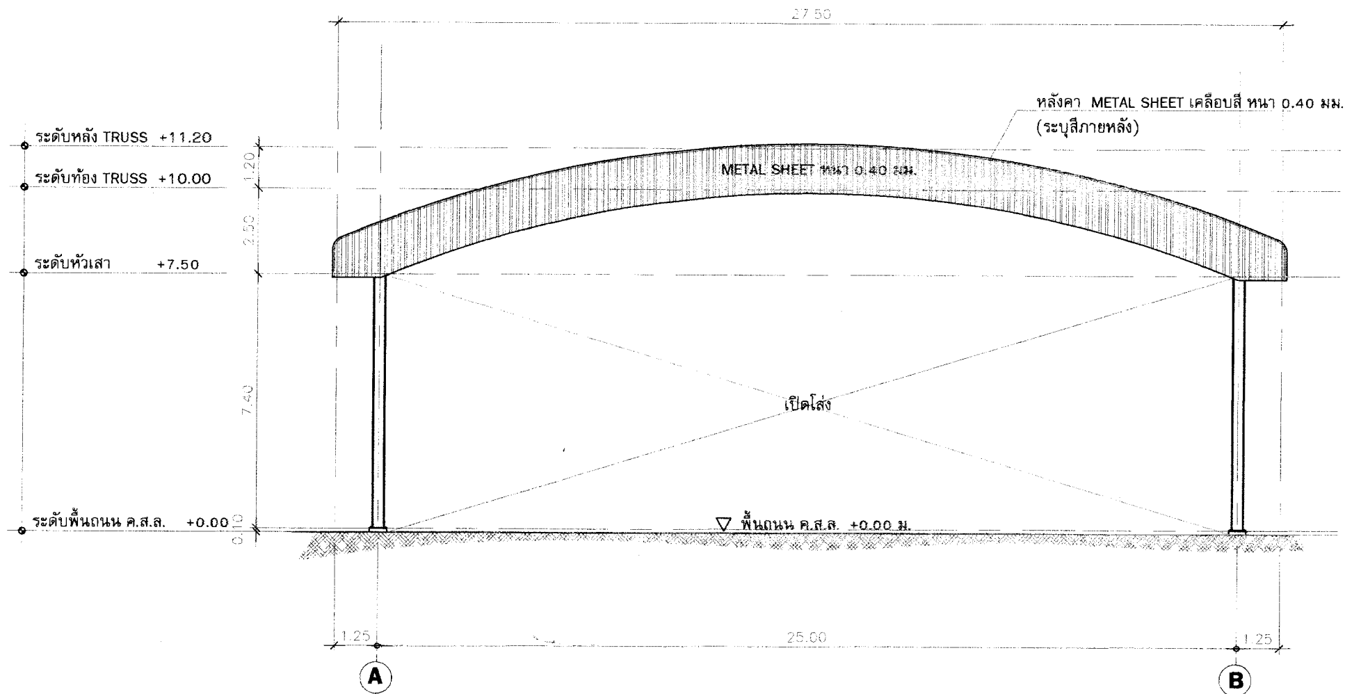
รูปด้าน 1 มาตรฐาน 1:100
