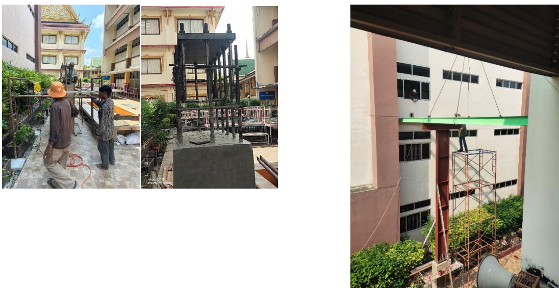
ภาพการวางระบบฐานรากและเสา
