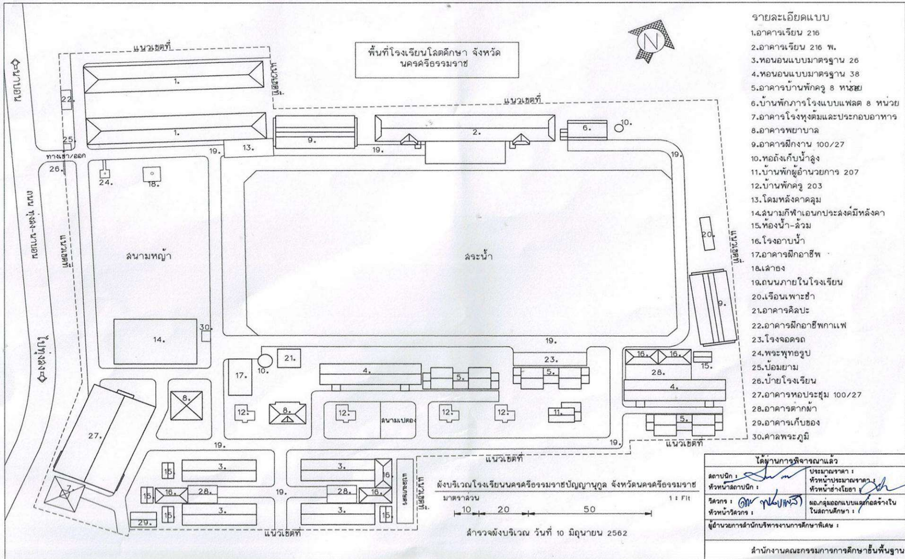
ภาพที่ ๑ แผนผังโรงเรียนนครศรีธรรมราชปัญญานุกูล จังหวัดนครศรีธรรมราช
